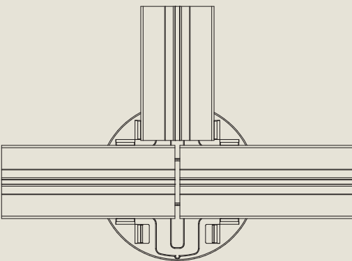
3 travetti di testa 3 front joists
